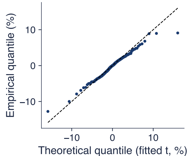
S&P 500 vs t(2.8)
