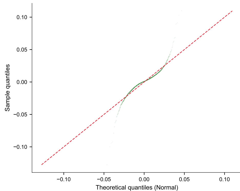
A. Normal QQ
