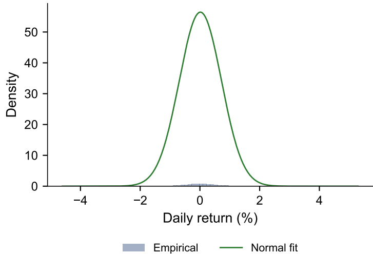
Histogram + Normal fit (kurt=6.09)
