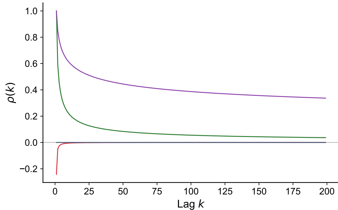
fGn ACF — linear scale
