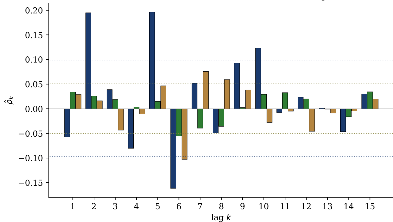
ACF BVB 2020--2025: BET, TLV, FP --- benzi 95% per serie
