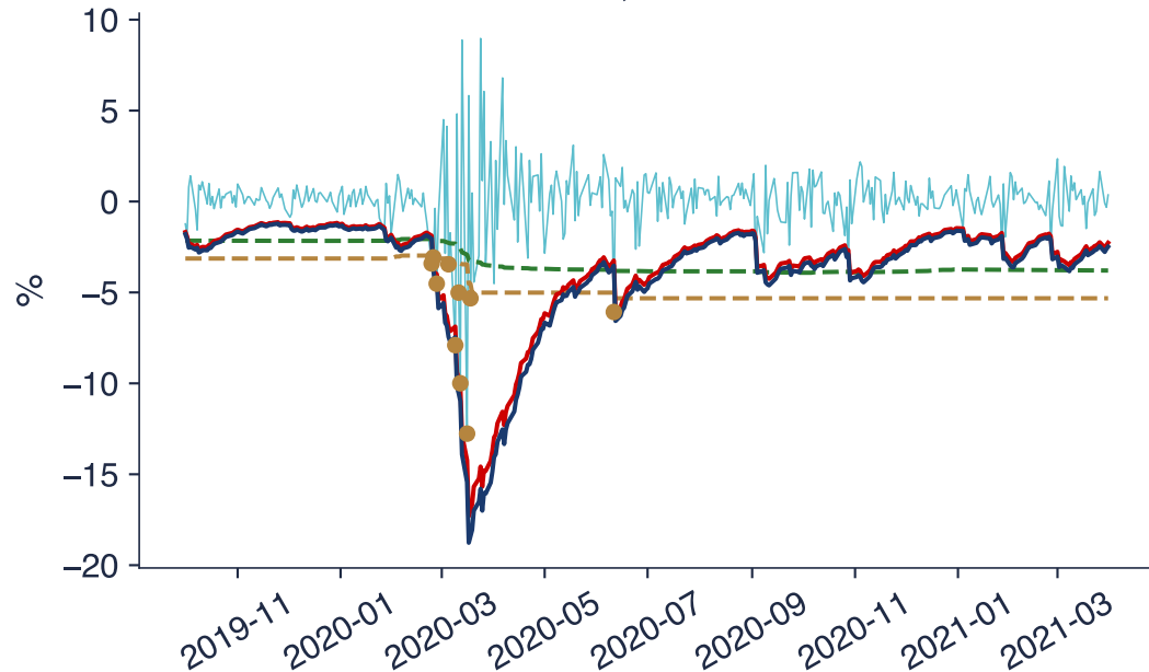
S&P 500, 2019-2021
