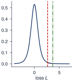
Student-t, 4 d.f., var. 1
