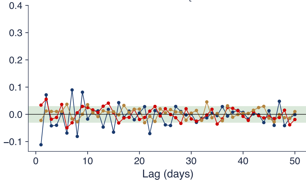
Returns r_t
