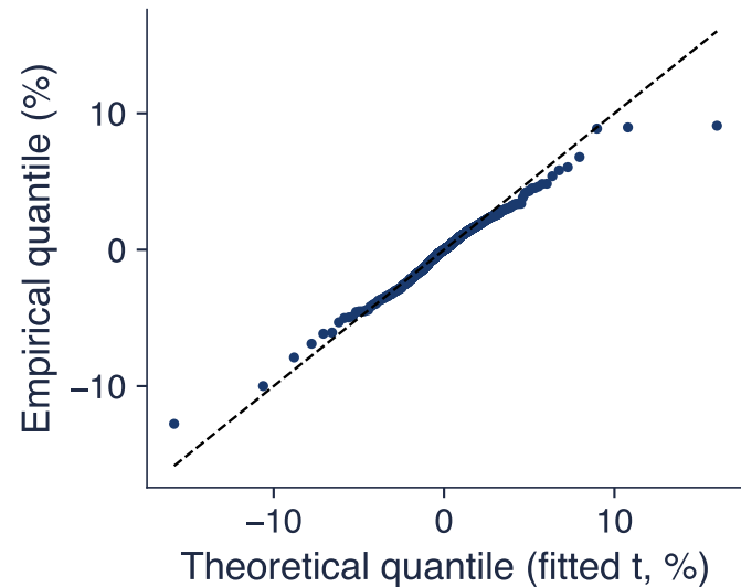
S&amp;P 500 vs t(2.8)
