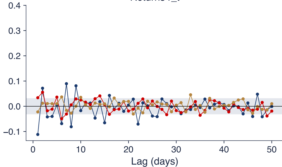
Returns r_t
