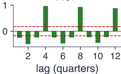
ACF
