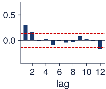
PACF
