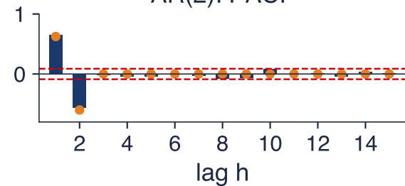
AR(2): PACF
