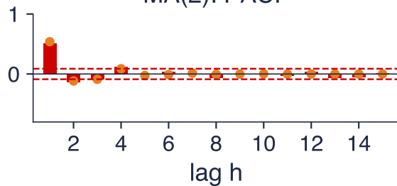
MA(2): PACF
