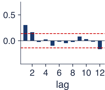
PACF
