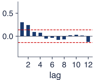
ACF
