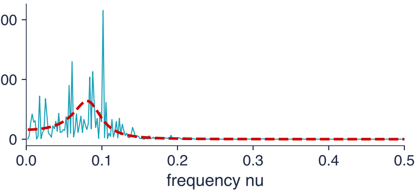
Raw periodogram
