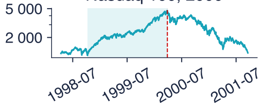
Nasdaq 100, 2000
