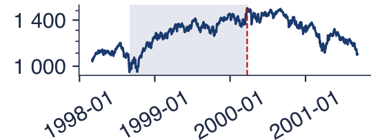
S&amp;P 500, 2000
