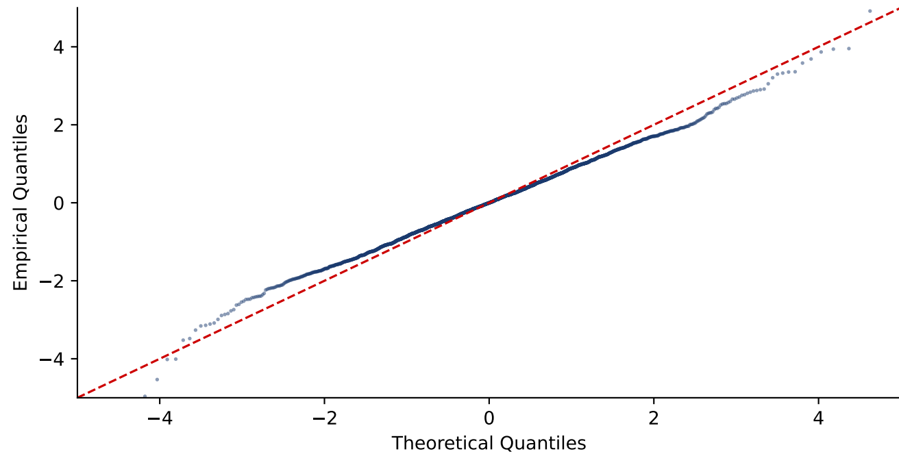
(d) Q-Q Plot (Student-t)
