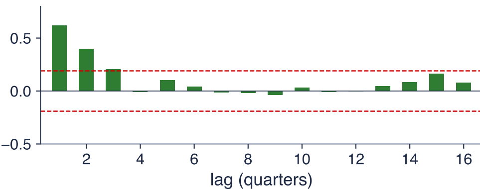
ACF
