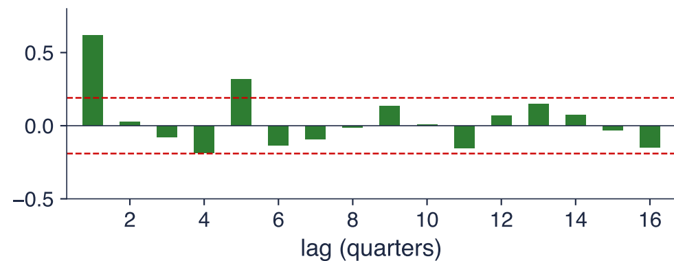
PACF
