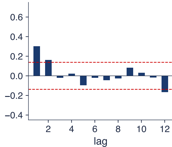
PACF
