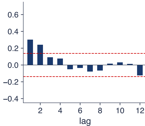
ACF
