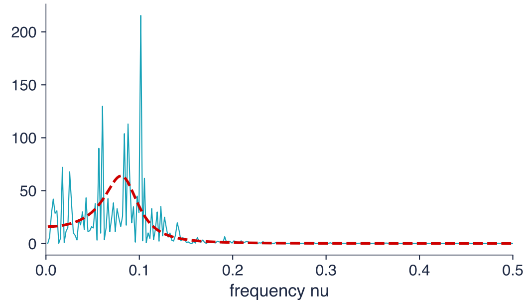
Raw periodogram
