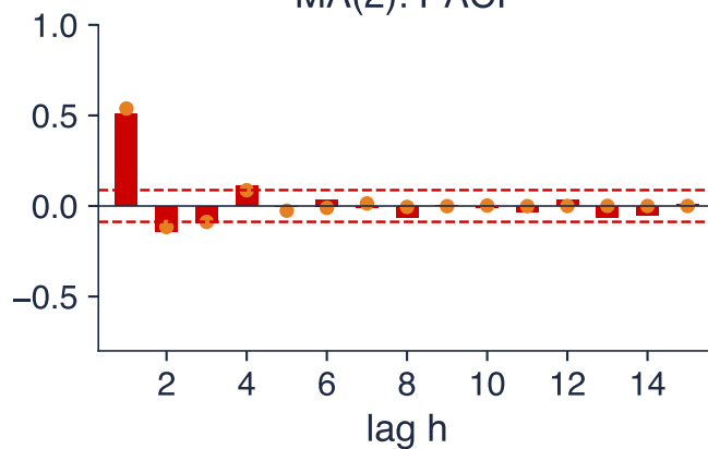
MA(2): PACF
