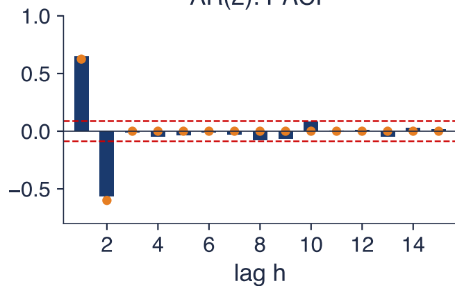
AR(2): PACF
