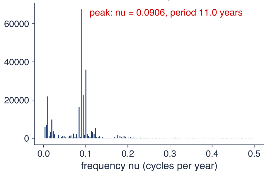
Raw periodogram
