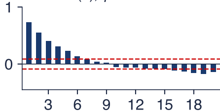
AR(1), \phi = 0.7 : ACF
