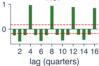
ACF
