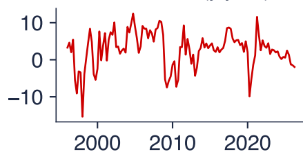
100 \Delta_4 \ln Y_t (y/y, %)
