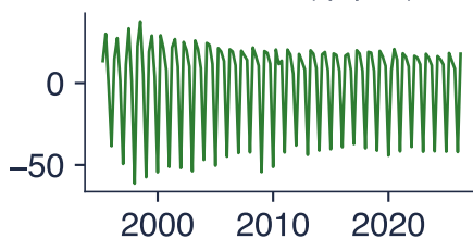
100 \Delta \ln Y_t (q/q, %)
