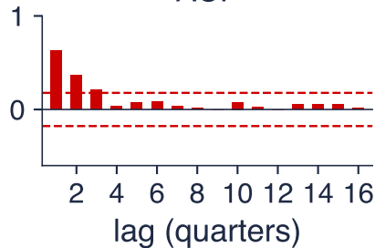
ACF
