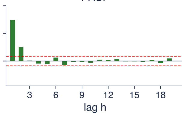
PACF
