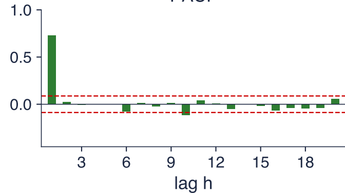
PACF
