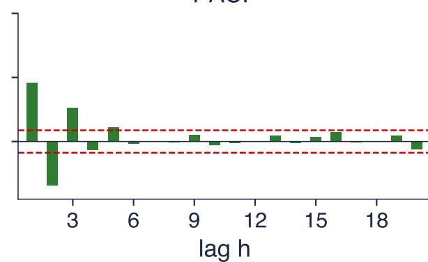
PACF
