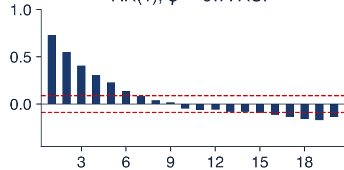
PACF
