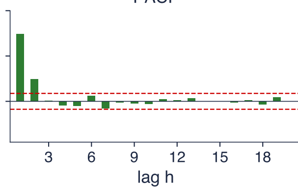
PACF
