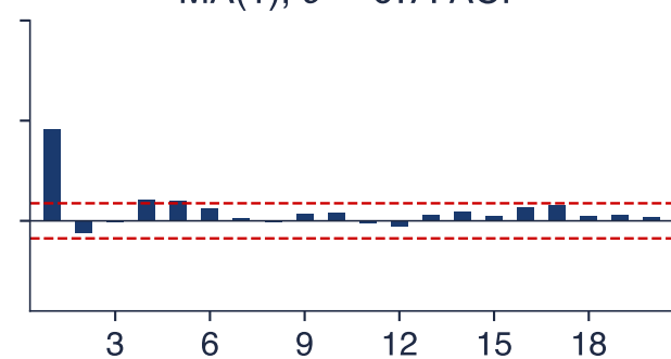
PACF
