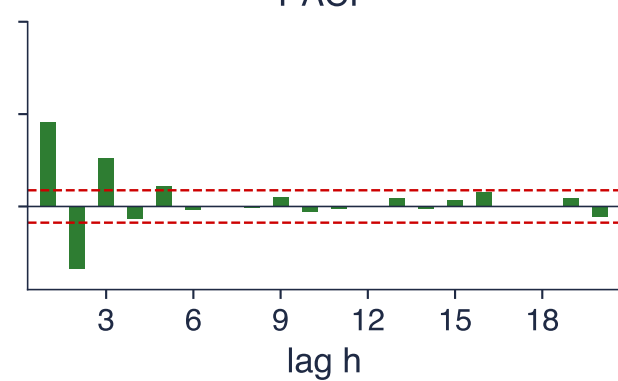
PACF
