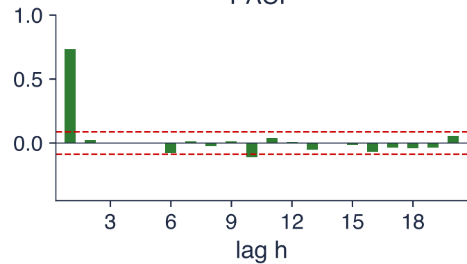
PACF
