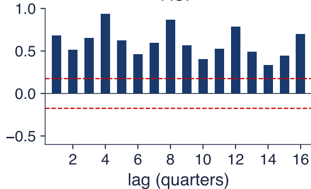
ACF
