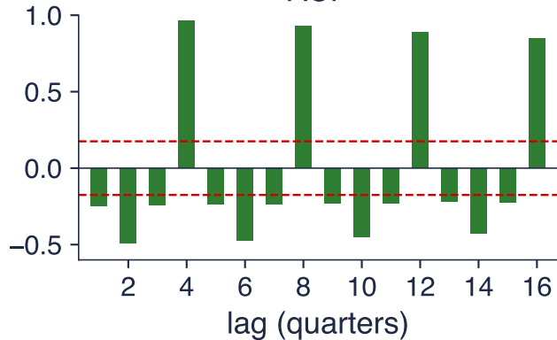
ACF
