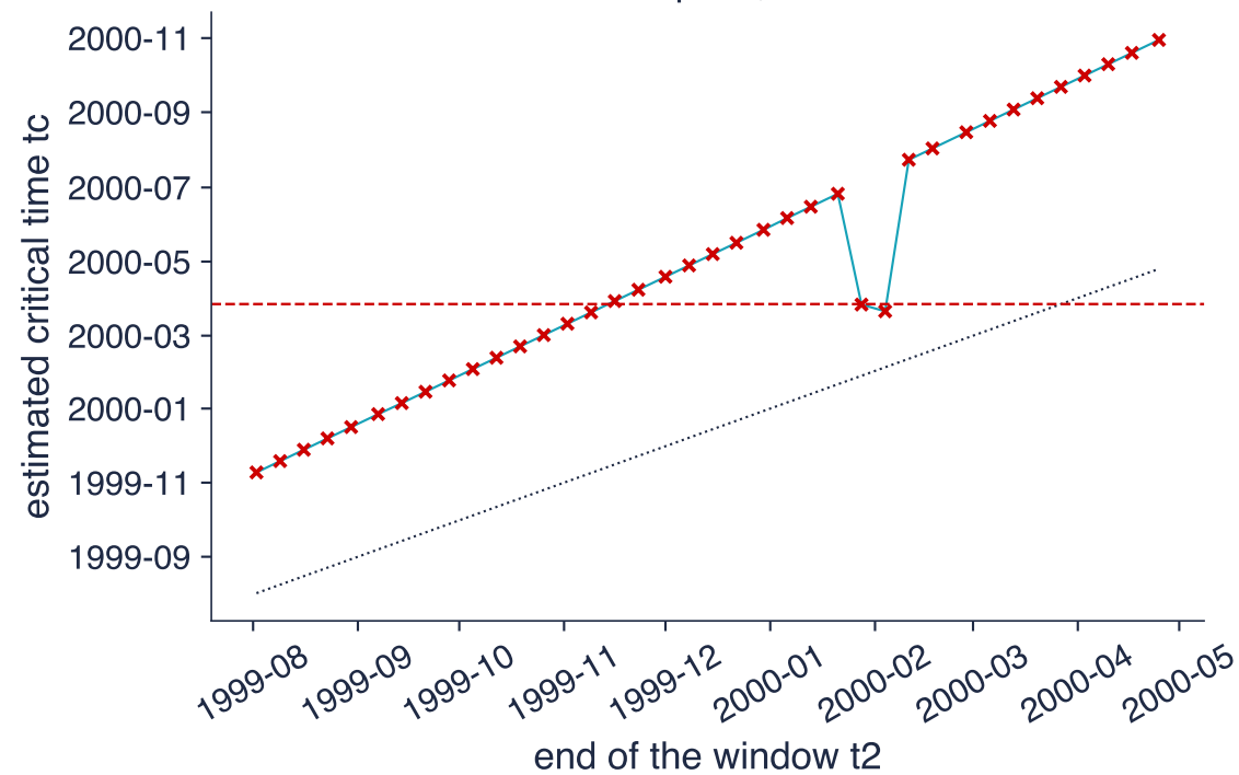
Nasdaq 100, 2000
