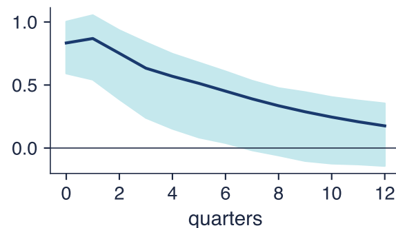
ROBOR 3M <- ROBOR 3M shock
