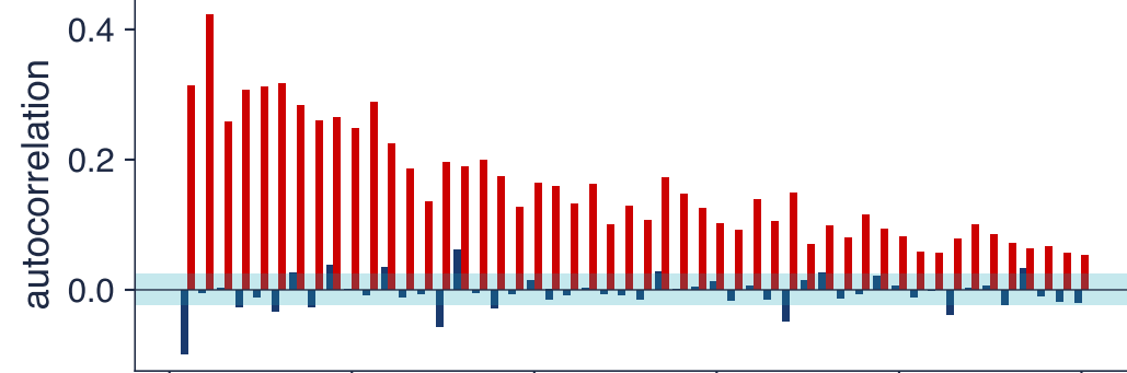
EUR/RON
