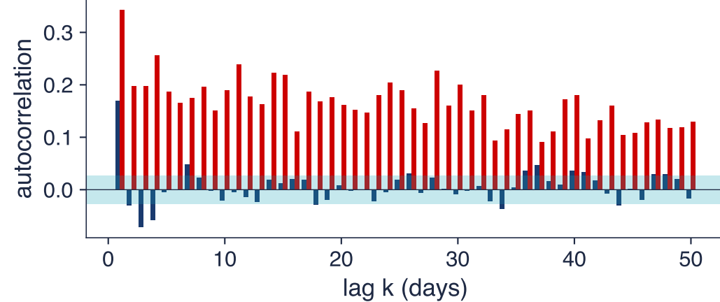
EUR/RON
