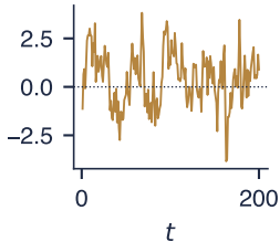
AR(1), \phi = 0.7
