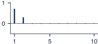
AR(2): PACF
