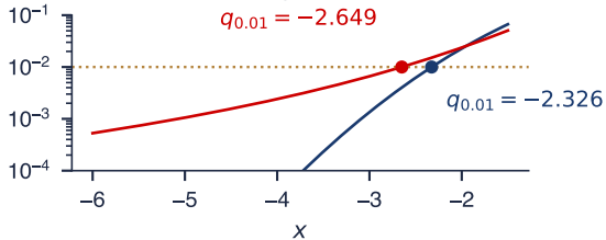
Left tail: P(z \leq x) , log scale
