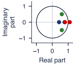
Eigenvalues
