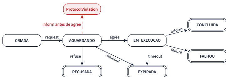
Figura 2: FSMs de delegação e do Approval Gate. Estados com borda dupla são finais; em vermelho, transições inválidas que viram testes negativos.
