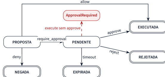
Figura 2: FSMs de delegação e do Approval Gate. Estados com borda dupla são finais; em vermelho, transições inválidas que viram testes negativos.
