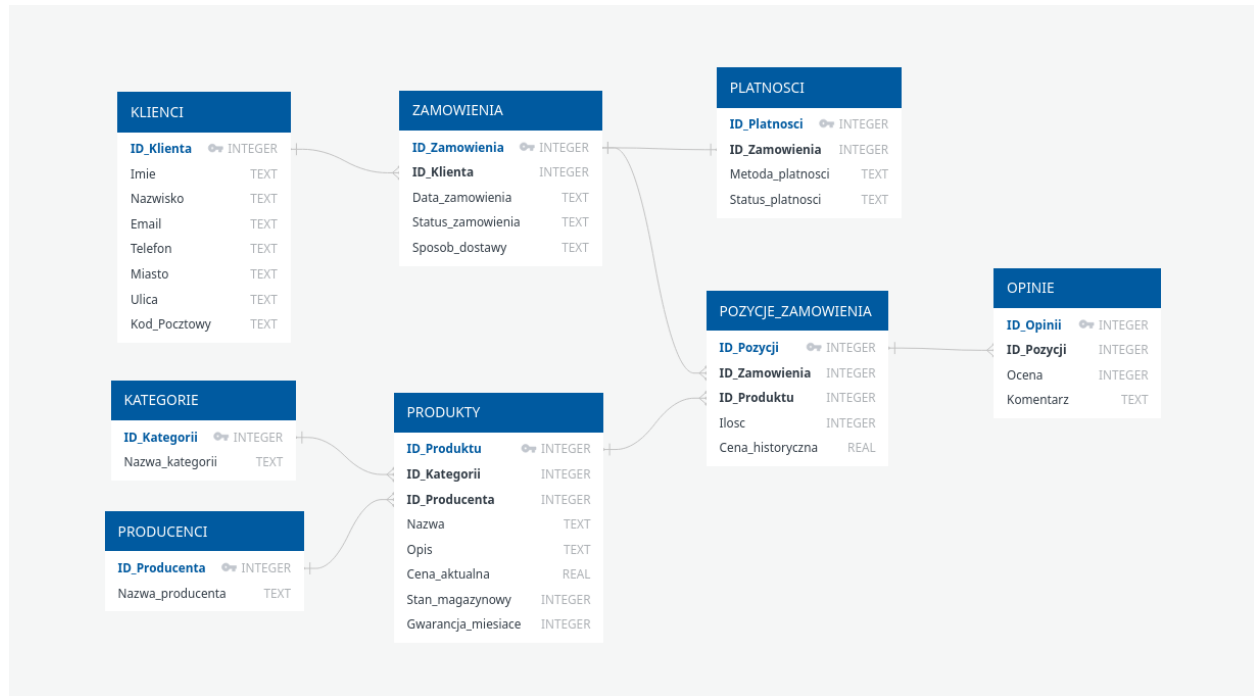
Rys. 3: Rysunek 3: Fizyczny schemat bazy danych opracowany dla silnika SQLite.
