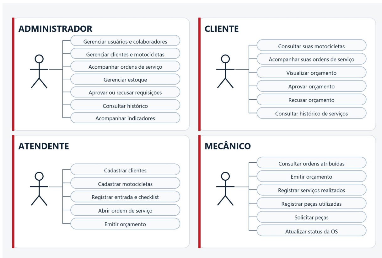
Figura 1 – Diagrama de Casos de Uso do Sistema Garagem 66
