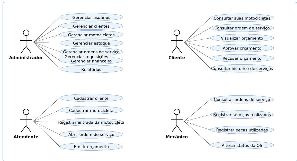
Figura 1 – Diagrama de Casos de Uso do Sistema Garagem 66
