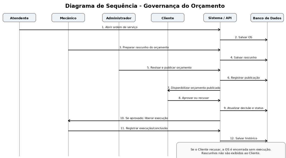
Figura 4 – Diagrama de Sequência do Sistema Garagem 66
