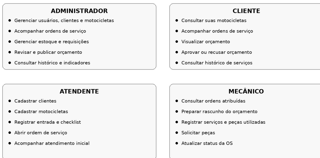
Figura 1 – Diagrama de Casos de Uso do Sistema Garagem 66
