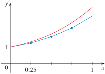
FIGURA 14 Aproximación de Euler con tamaño de paso 0.25
