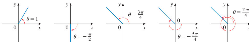
FIGURA 5 Ángulos en posición estándar
