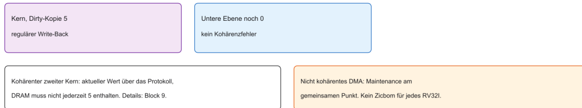
Abbildung 11: Dirty-Kopie 5 bei altem Wert 0 ist zunächst Write-Back, kein Kohärenzfehler. Kohärente Leser und nicht kohärentes DMA sind getrennte Fälle.
