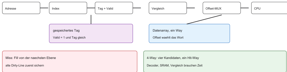
Abbildung 8: Index öffnet das Set, Tag und Valid vergleichen, Offset wählt das Wort, Daten gehen zur CPU.
