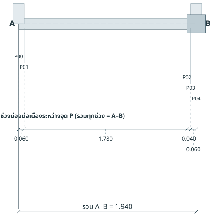
ผังขยายตามแกน A→B / 1:25
