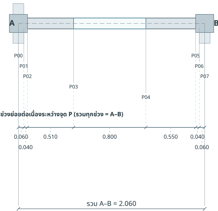
ผังขยายตามแกน A→B / 1:25
