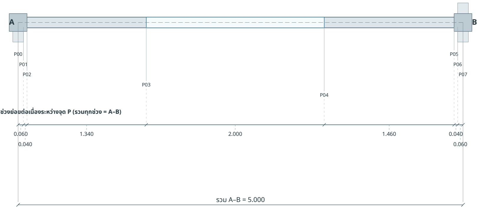
ผังขยายตามแกน A→B / 1:25
