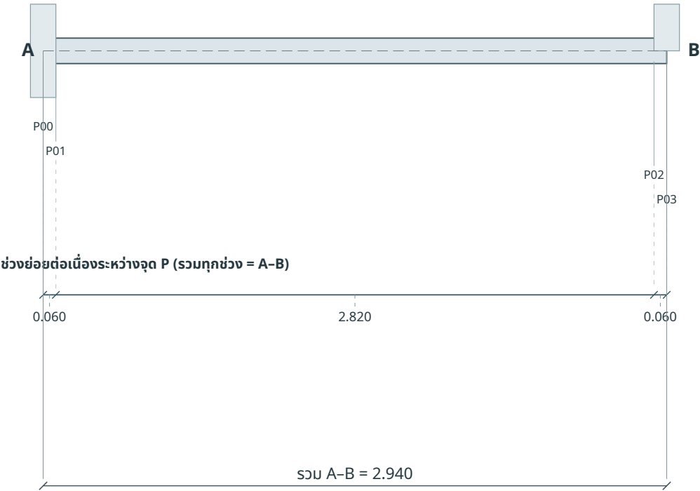
ผังขยายตามแกน A→B / 1:25
