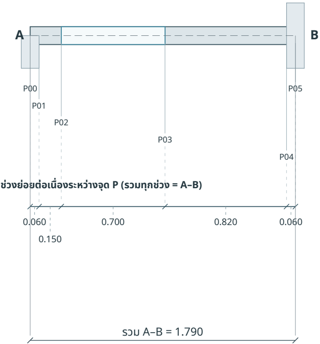
ผังขยายตามแกน A→B / 1:25
