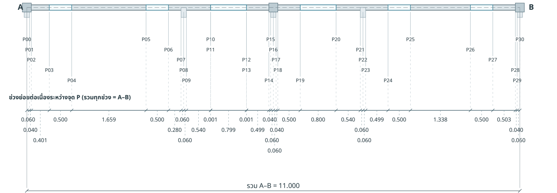
รูปด้านคลี่ A→B / 1:50
