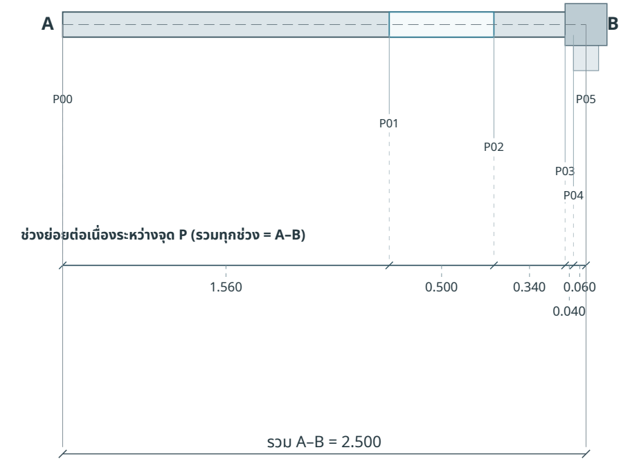
ผังขยายตามแกน A→B / 1:25
