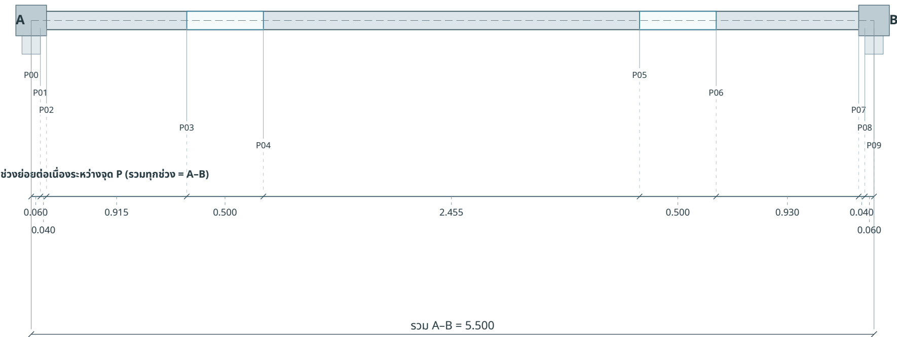
ผังขยายตามแกน A→B / 1:25
