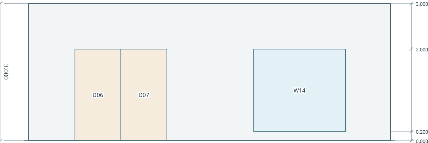
รูปด้านคลี่ A→B / 1:50
