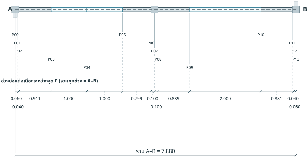
ผังขยายตามแกน A→B / 1:50
