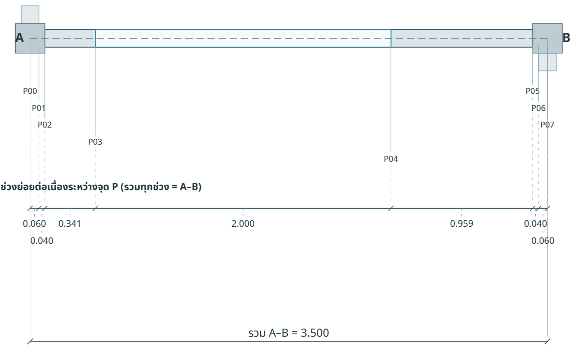
ผังขยายตามแกน A→B / 1:25
