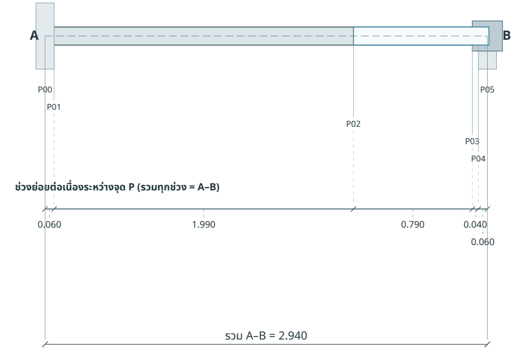
ผังขยายตามแกน A→B / 1:25
