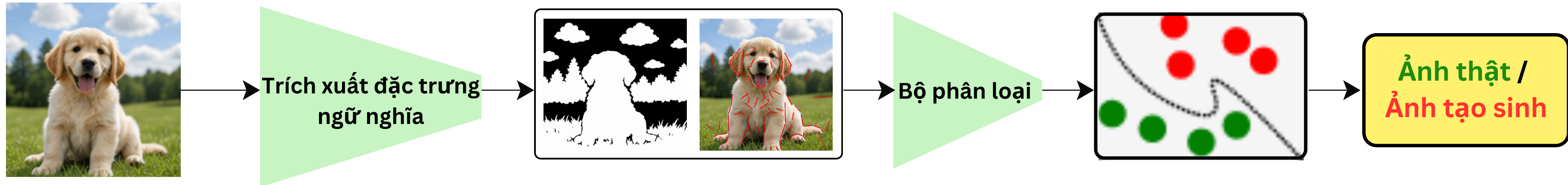
b) Các phương pháp phân loại dựa trên đặc trưng ngữ nghĩa
