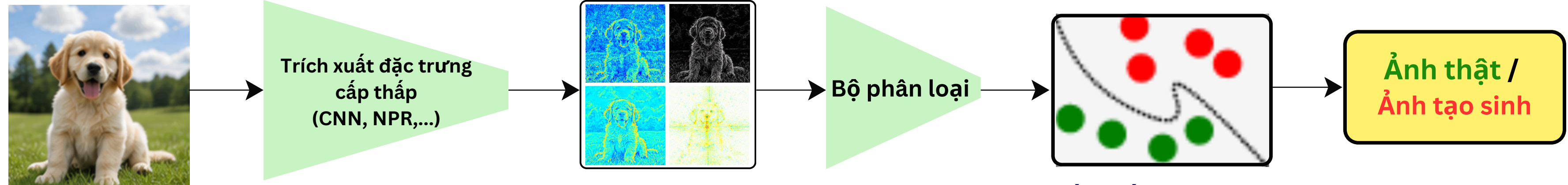
a) Các phương pháp phân loại dựa trên đặc trưng cấp thấp
