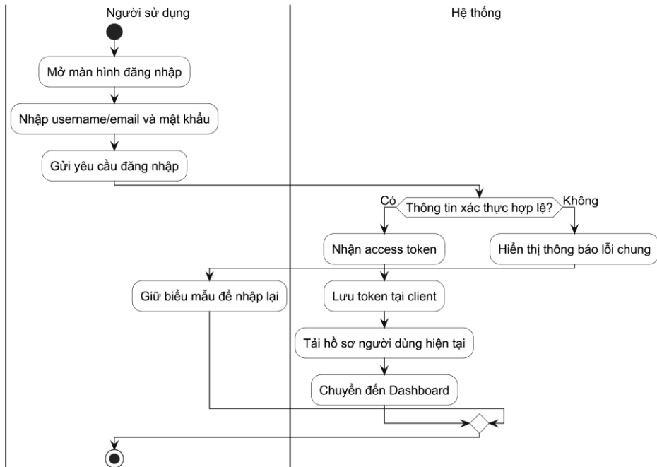
UC002 — ACTIVITY DIAGRAM ĐĂNG NHẬP
