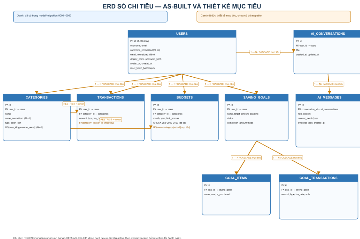
Hình 24. ERD as-built và thiết kế mục tiêu
