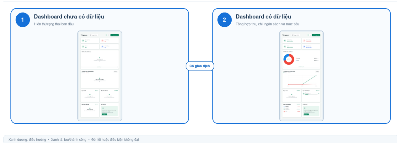
Hình 5. Luồng Dashboard
