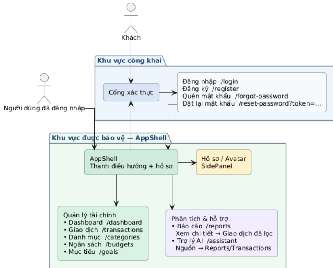
Hình 1. Luồng sử dụng tổng thể của ứng dụng
