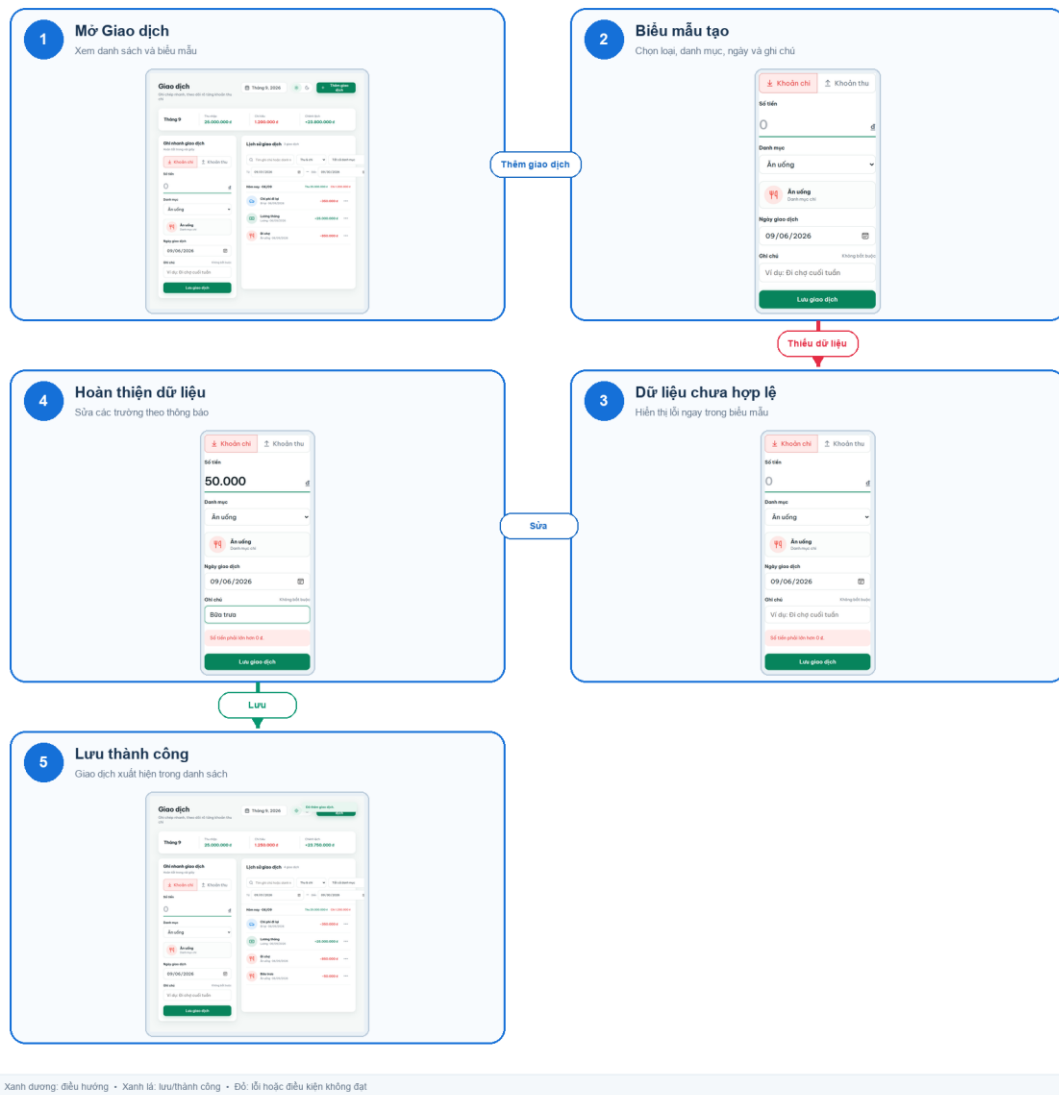
Hình 8. Luồng tạo giao dịch
