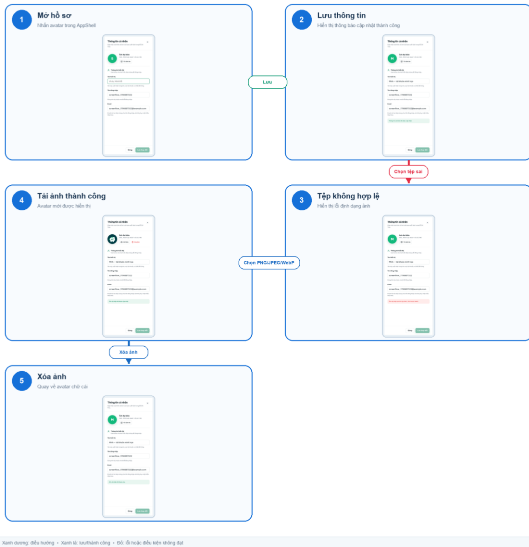
Hình 6. Luồng quản lý hồ sơ và ảnh đại diện
