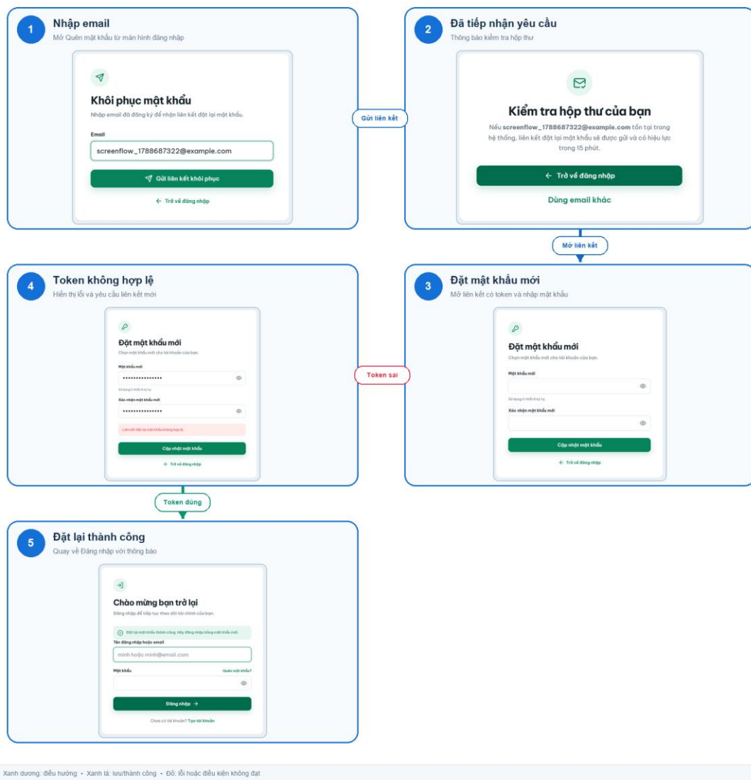
Hình 4. Luồng khôi phục mật khẩu
