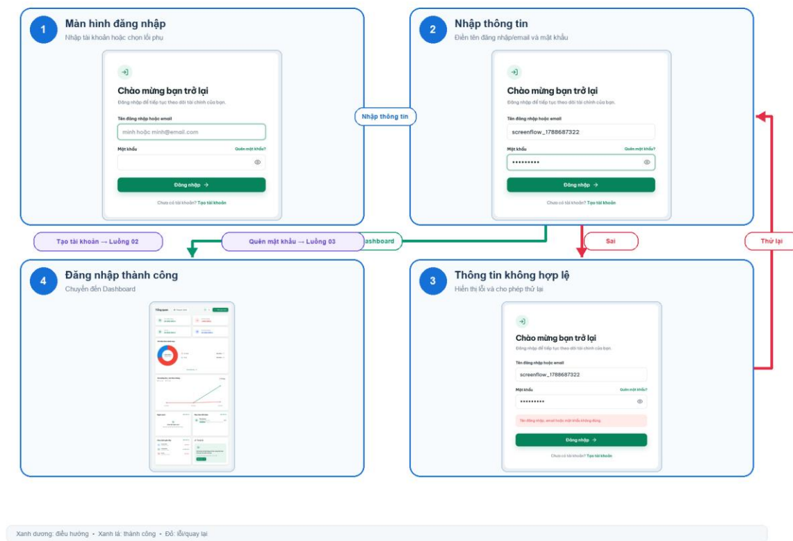
Hình 3. Luồng đăng nhập
