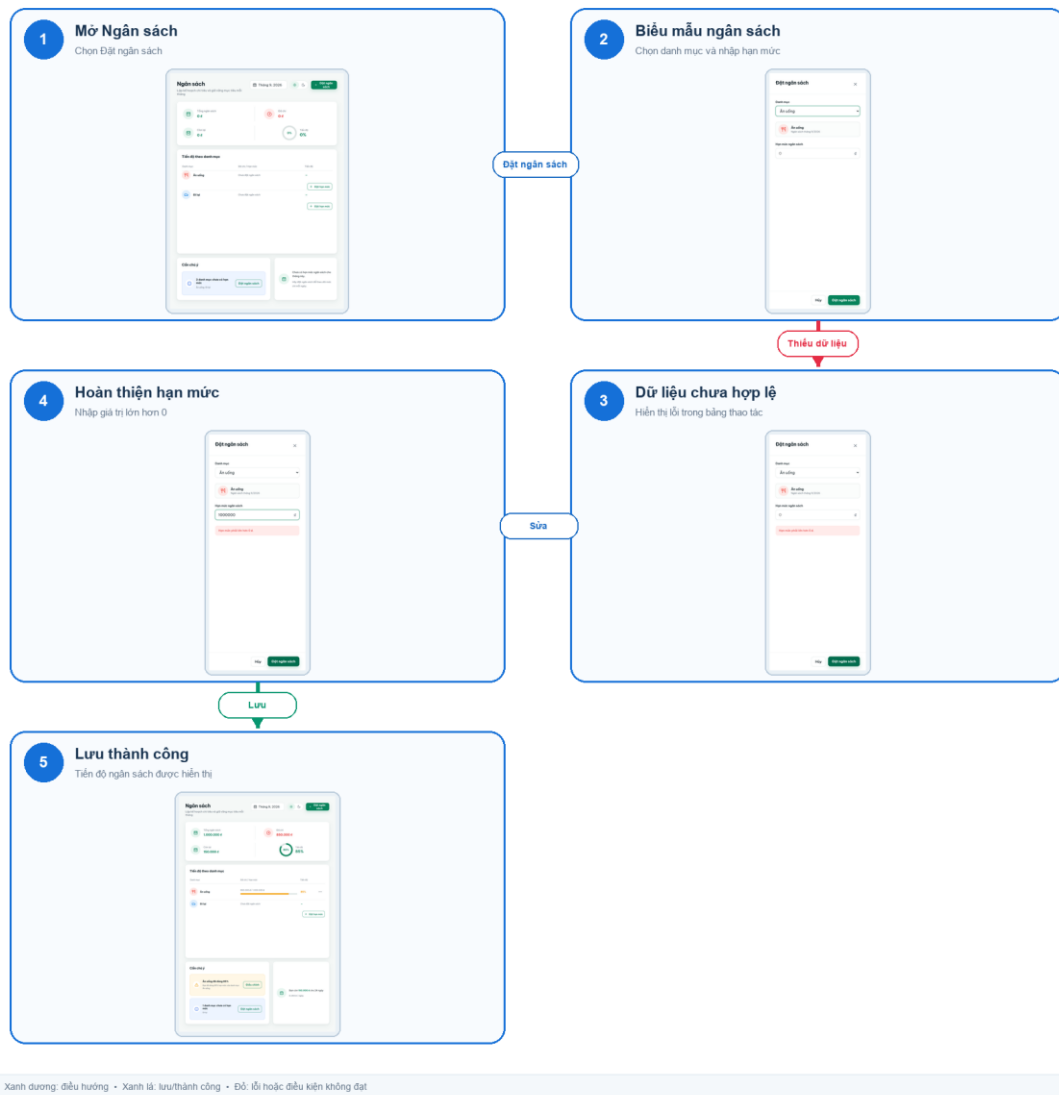
Hình 9. Luồng đặt ngân sách
