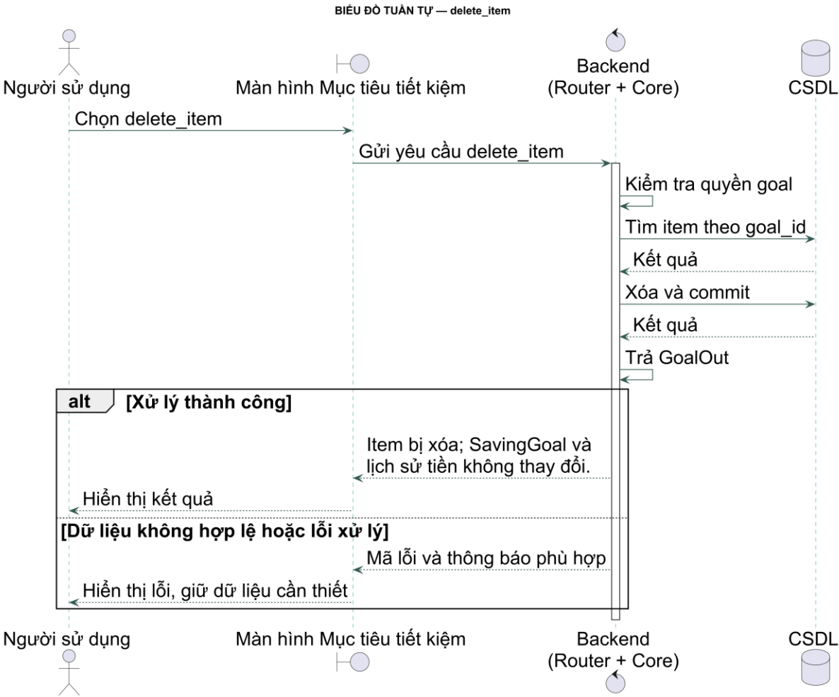
Biểu đồ tuần tự – delete_item
