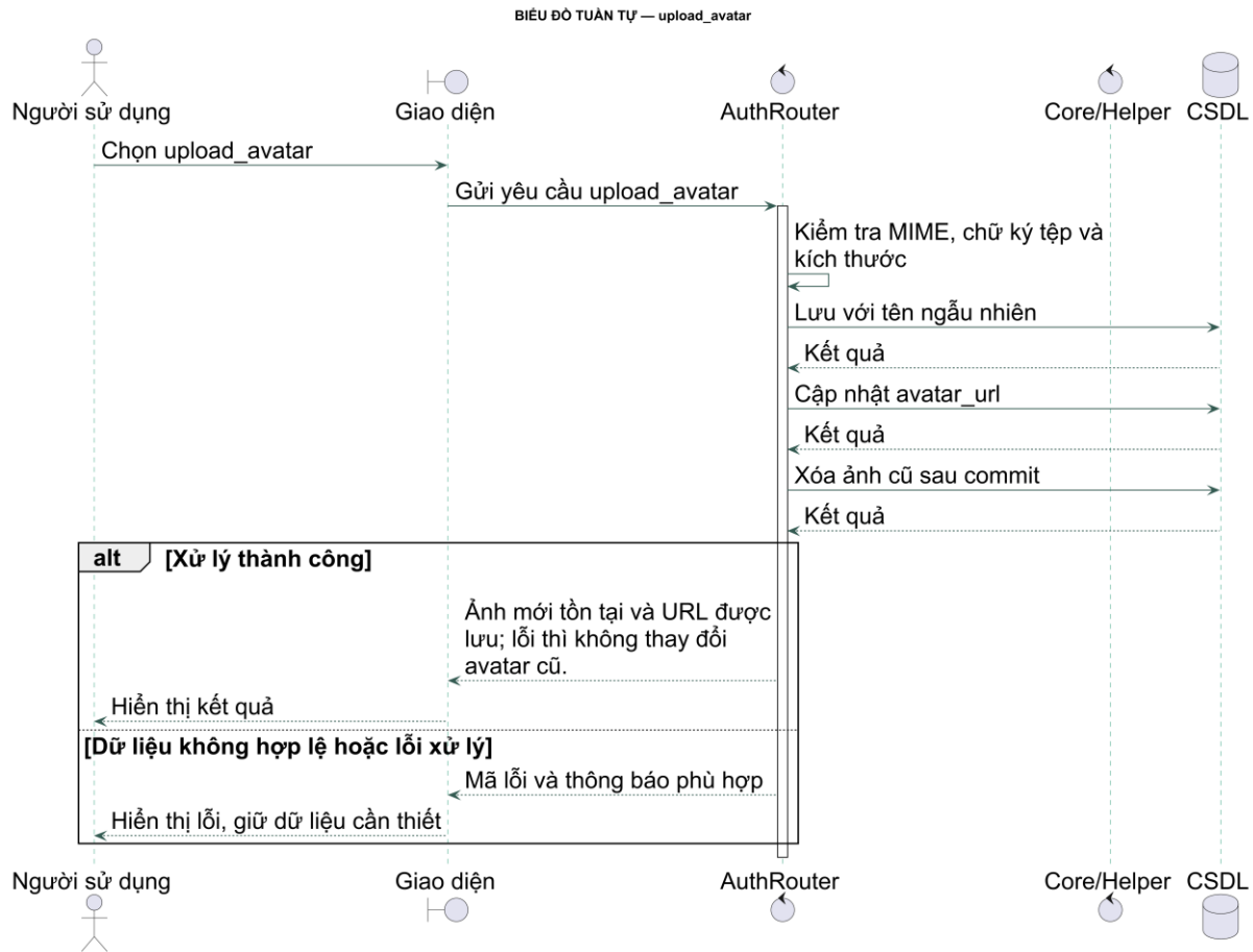
Biểu đồ tuần tự – upload_avatar
