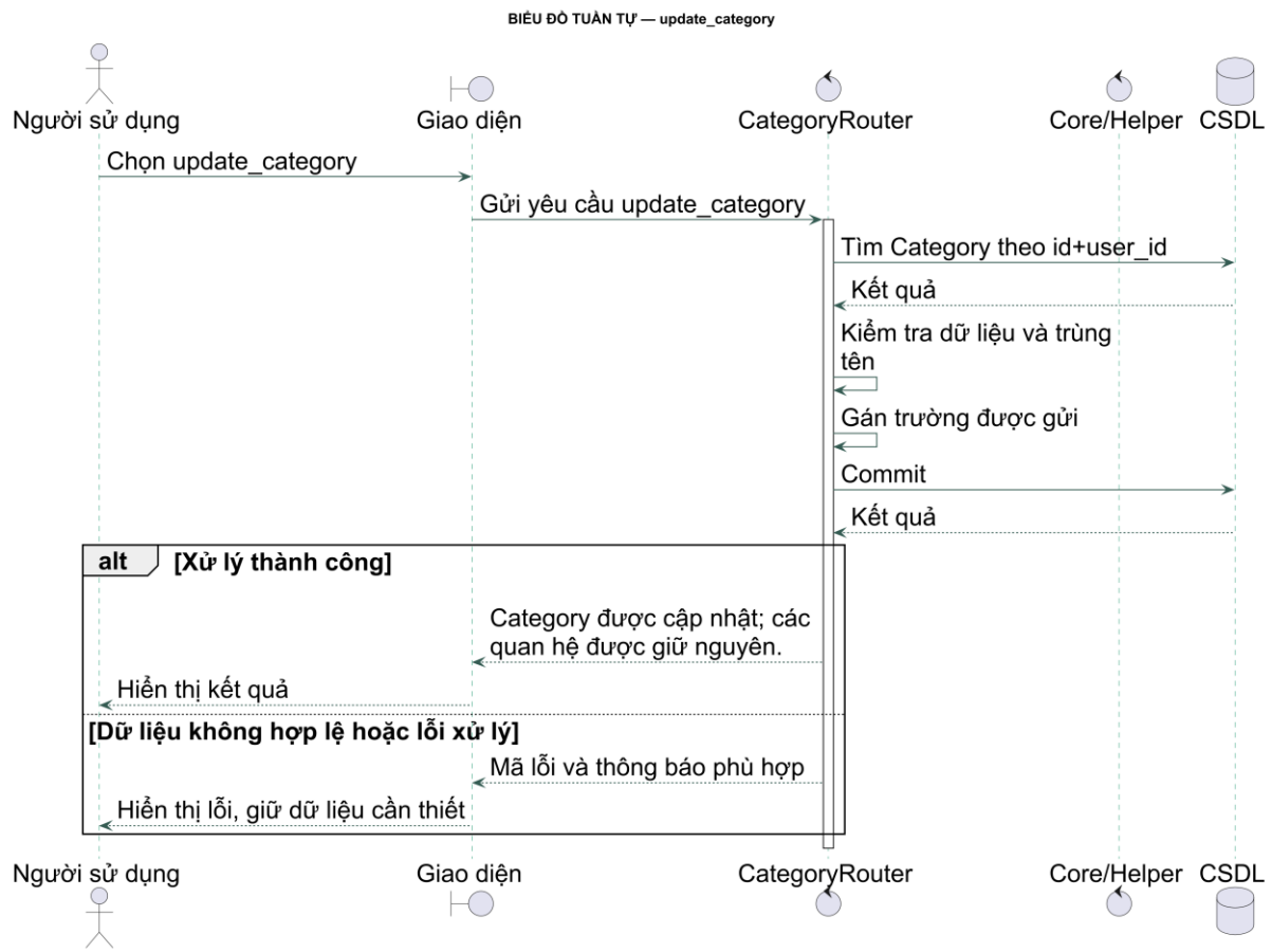
Biểu đồ tuần tự – update_category
