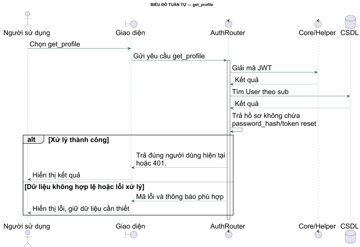
Biểu đồ tuần tự – get_profile
