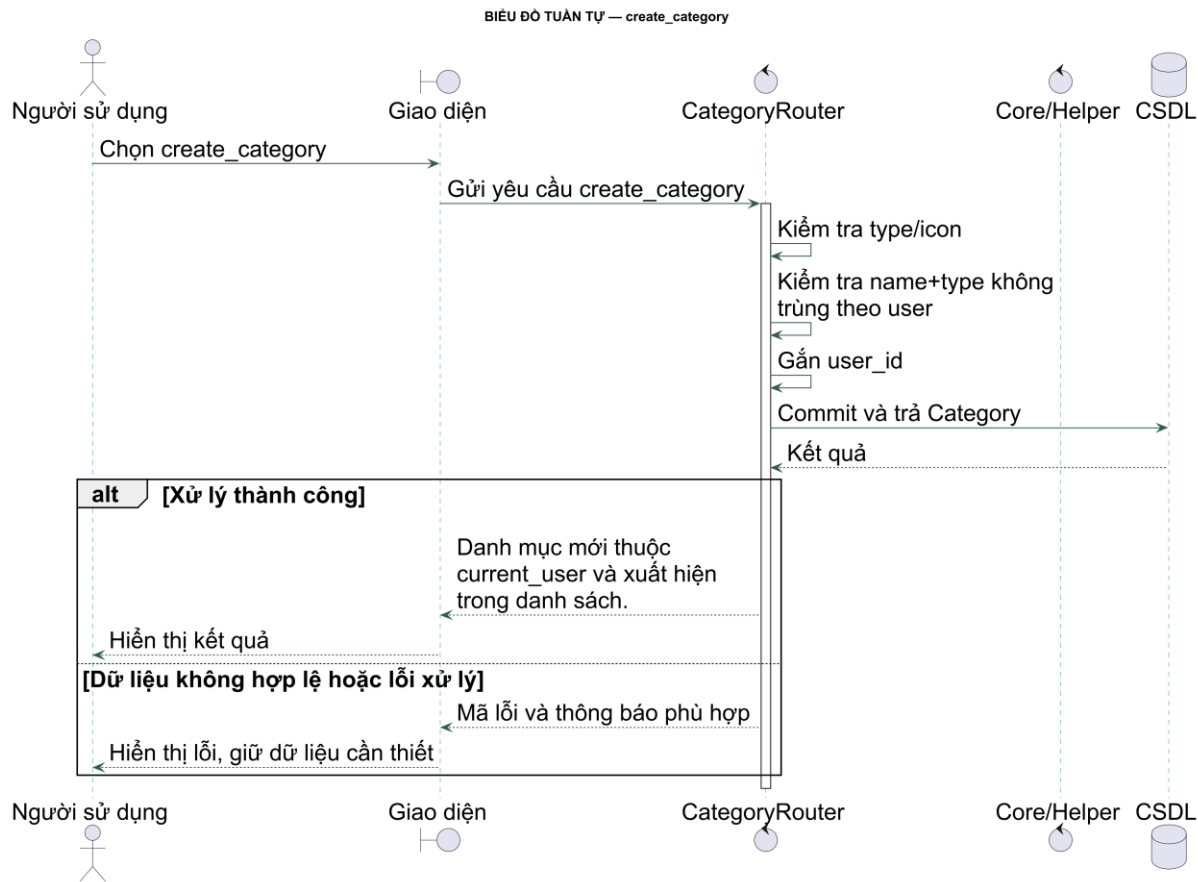
Biểu đồ tuần tự – create_category
