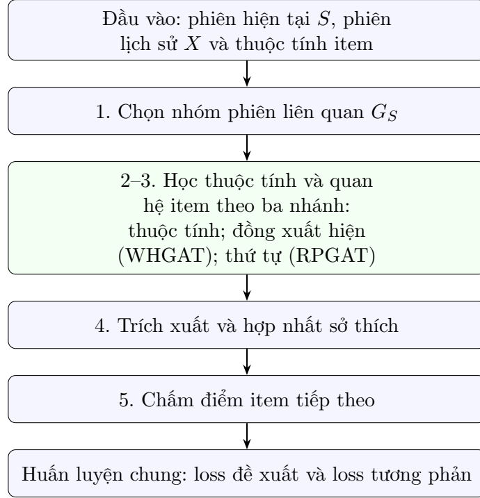
Hình 1: Sơ đồ khái quát các thành phần của MLEUP, dựng lại theo mô tả trong bài báo.
