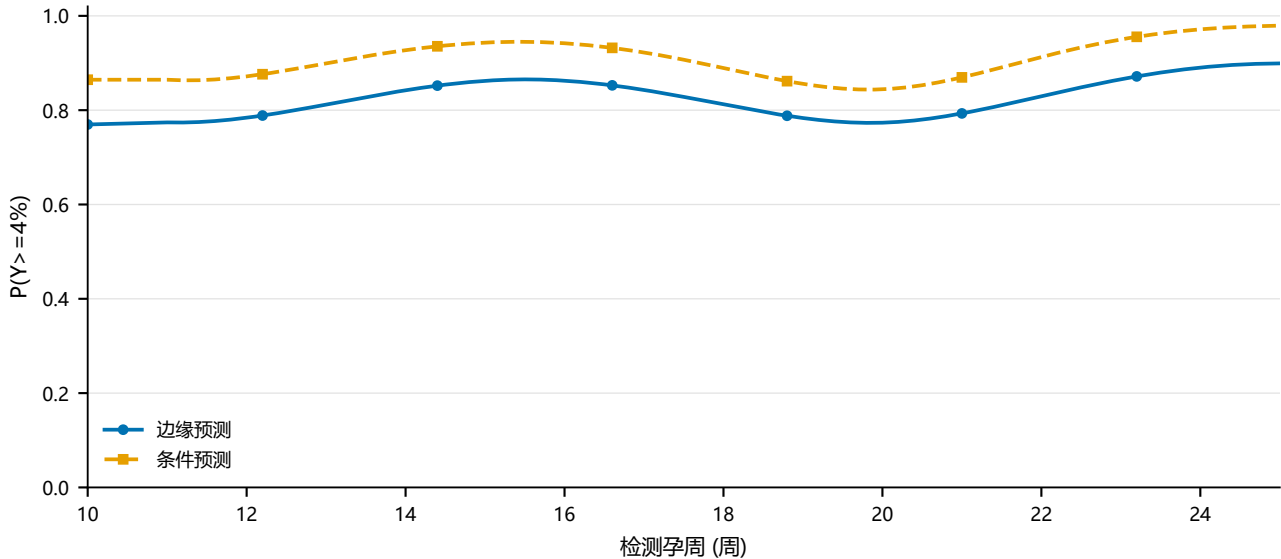
个体随机效应积分的影响
